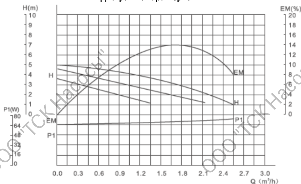
Диаграмма характеристик
