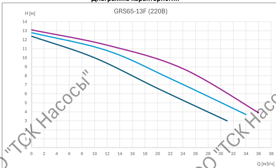
Диаграмма характеристик
