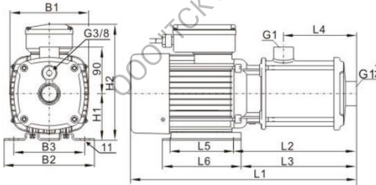
Габаритный чертёж
