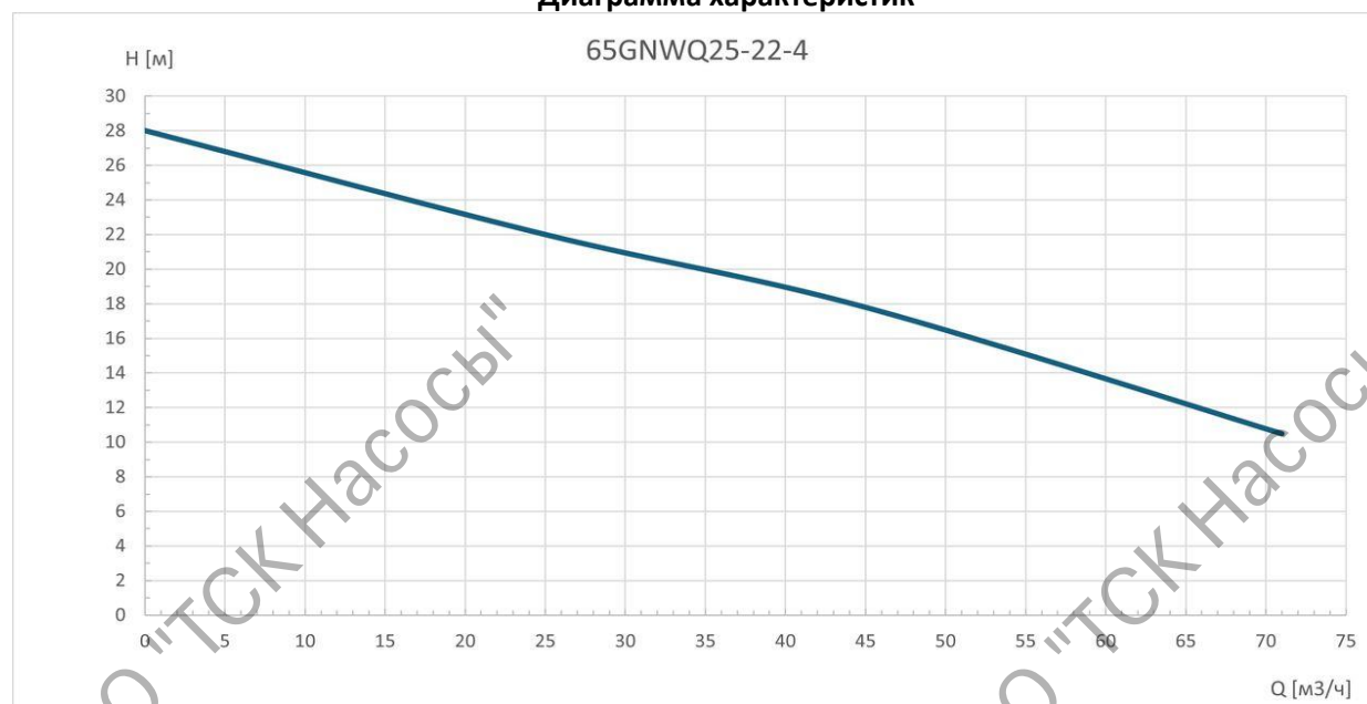
Диаграмма характеристик
