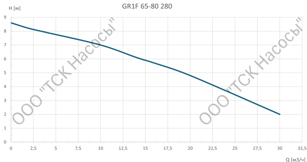
Диаграмма характеристик
