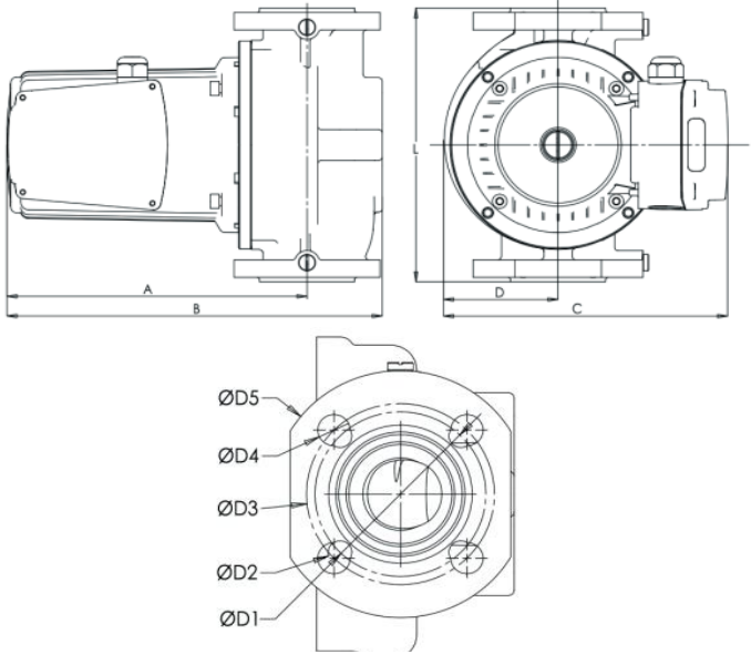
Габаритный чертёж
