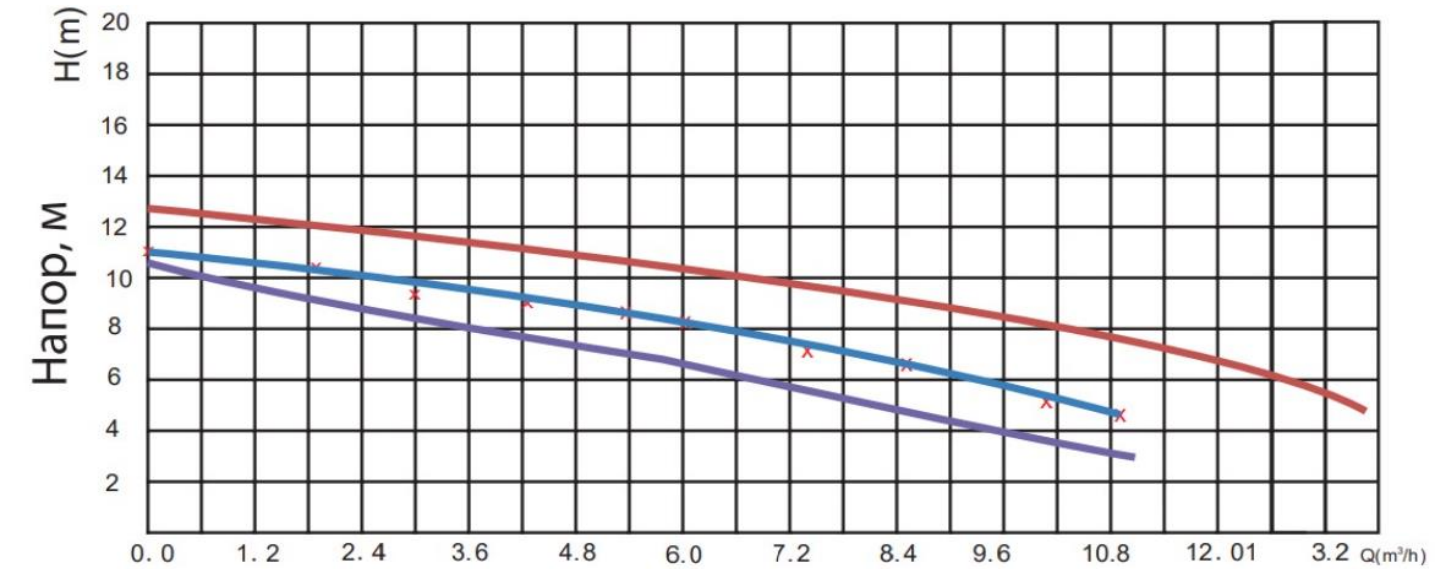
Диаграмма характеристик
