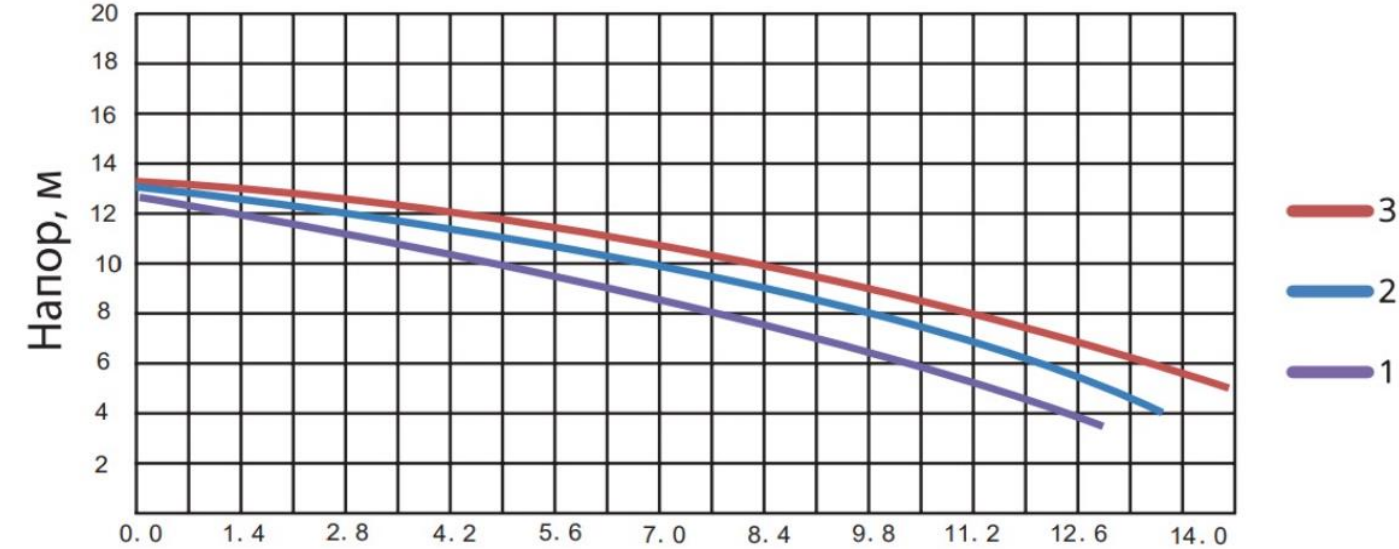
Диаграмма характеристик
