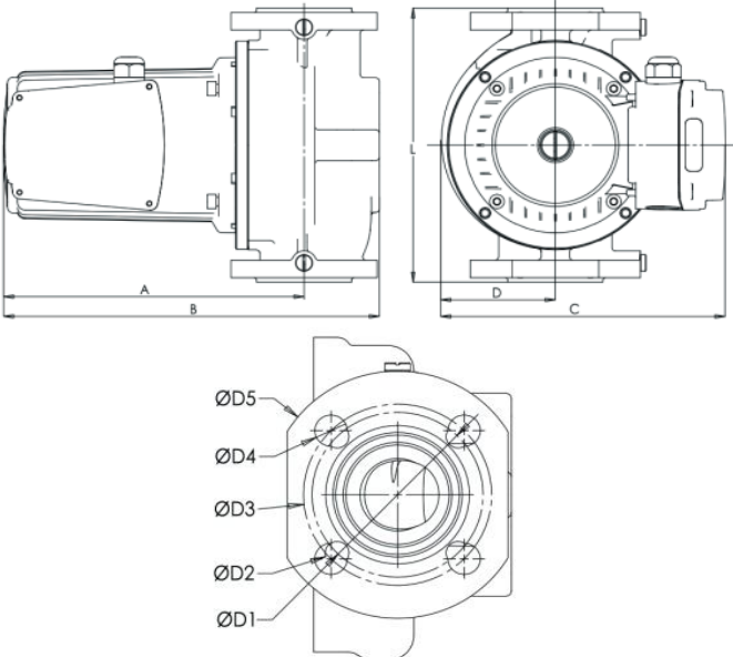
Габаритный чертёж
