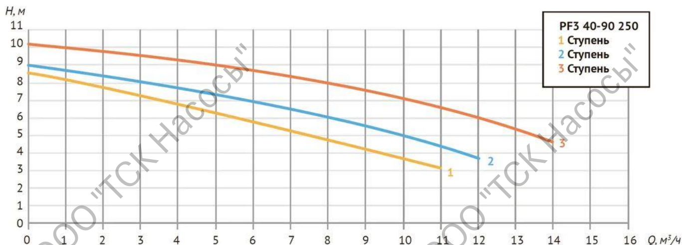
Диаграмма характеристик
