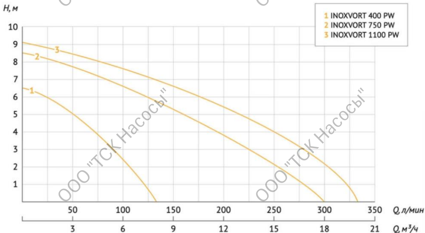
Диаграмма характеристик
