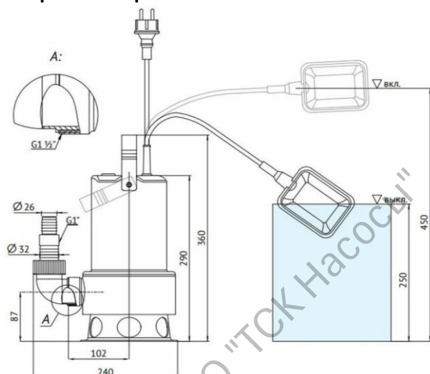
Габаритный чертёж
