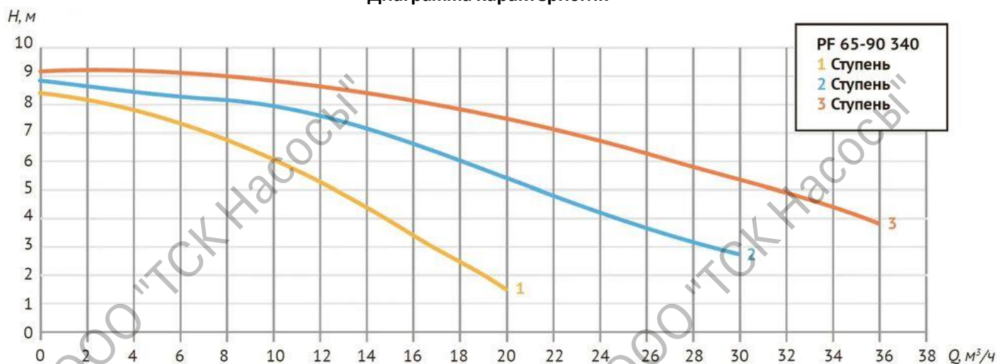
Диаграмма характеристик
