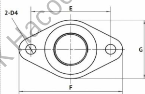
Выходной патрубок
