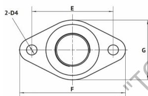
Входной патрубок
