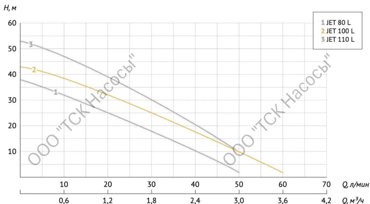
Диаграмма характеристики
