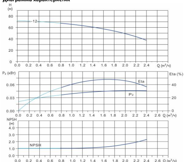
Диаграмма характеристик
