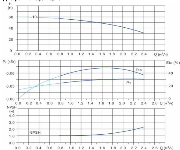
Диаграмма характеристик
