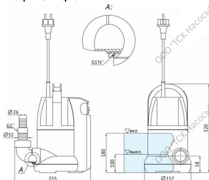
Габаритный чертёж
