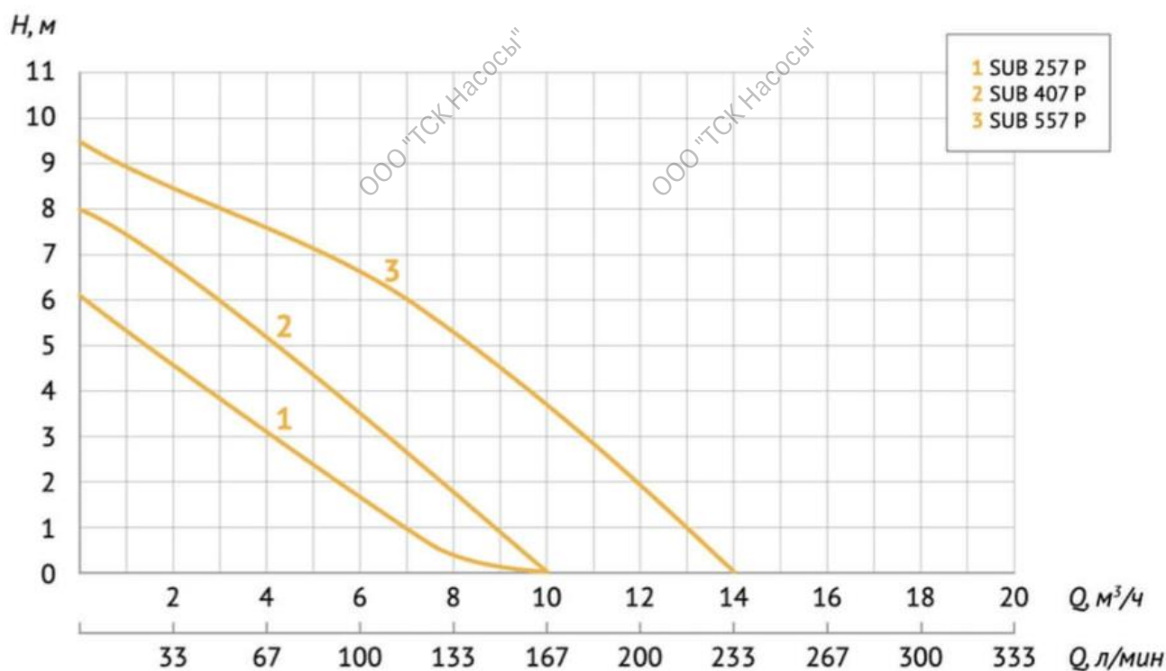
Диаграмма характеристик
