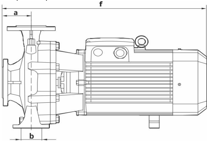
Габаритный чертёж
