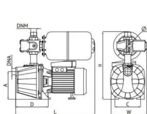
Гидроаккумулятор 5 л
