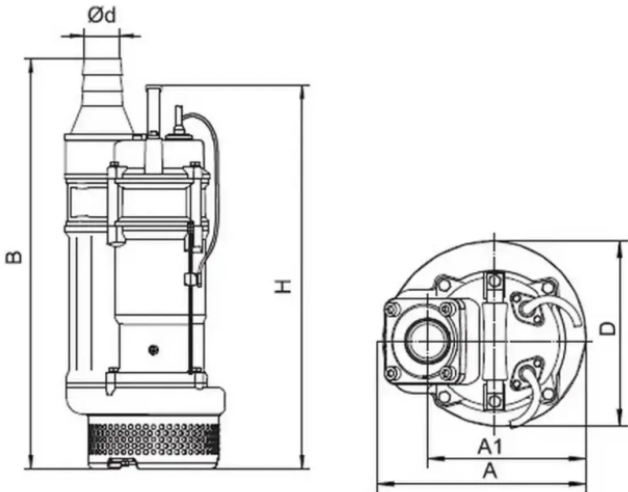
Рисунок 2 – Габаритные и присоединительные размеры насосов серии USPA
