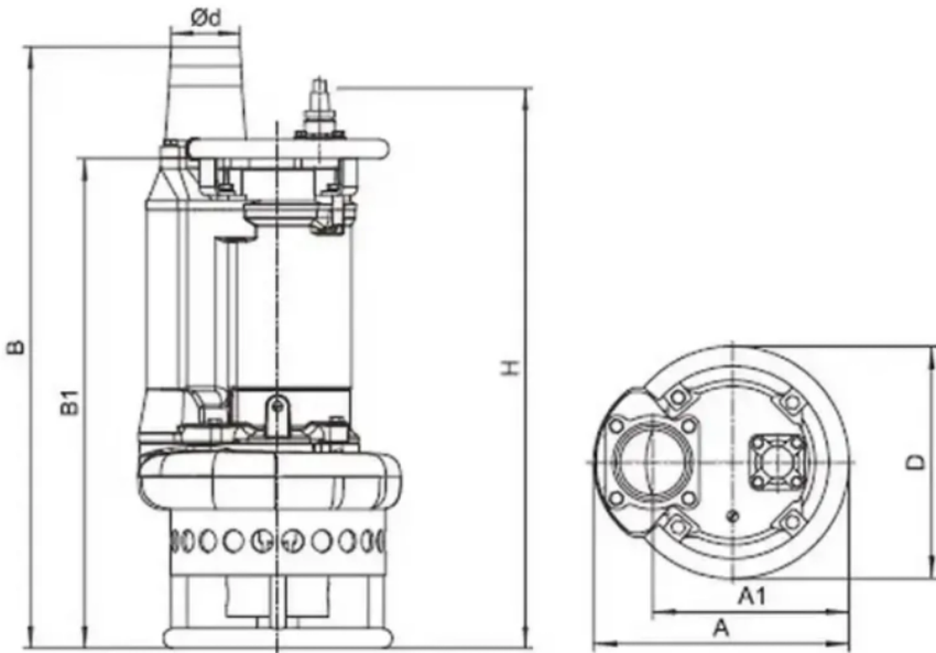
Рисунок 3 – Габаритные и присоединительные размеры насосов серии USP4A
