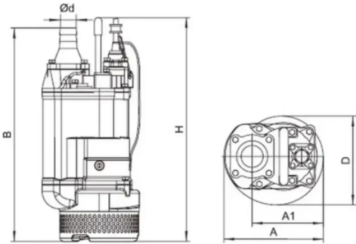
Рисунок 1 – Габаритные и присоединительные размеры насосов серии USP
