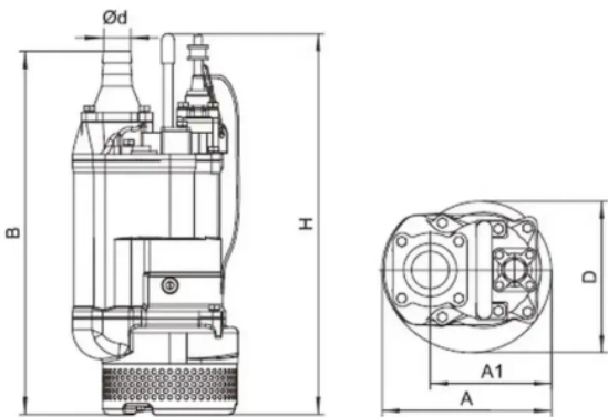
Рисунок 1 – Габаритные и присоединительный размеры насосов серии USP
