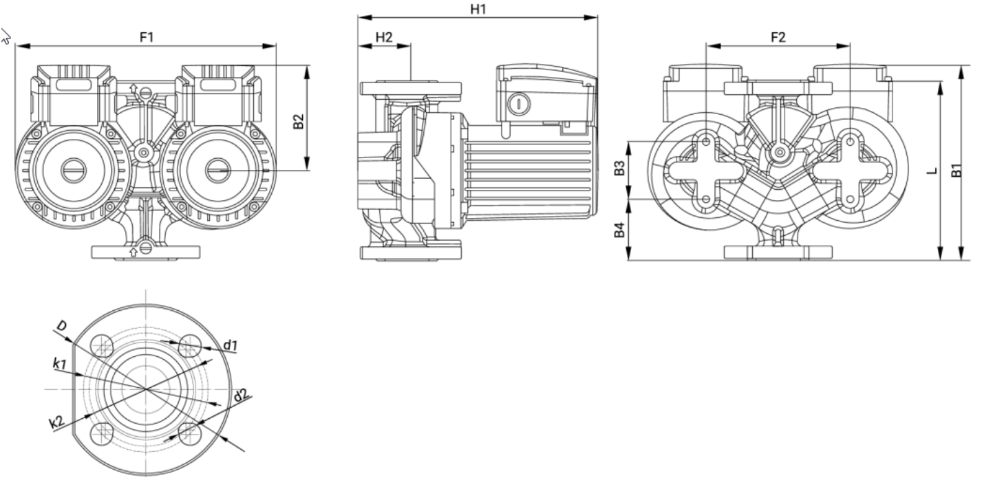
Габаритные размеры, мм
