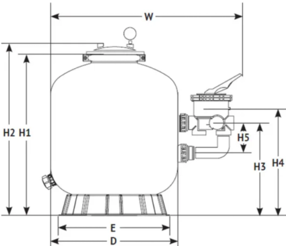
Габаритные и присоединительные размеры
