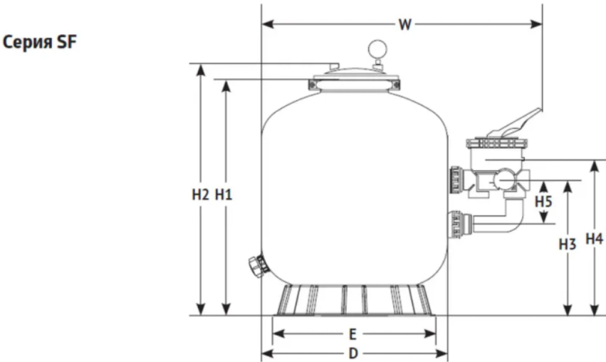
Габаритные и присоединительные размеры
